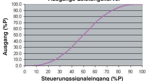
Phasenwinkel-Befehlssignaleingang zu Ausgangs-Leistungskurve.
